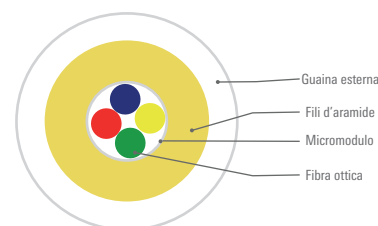
Taglio del cavo a 4 fibre
