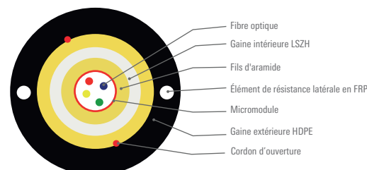
Coupe du câble version 4 fibres
