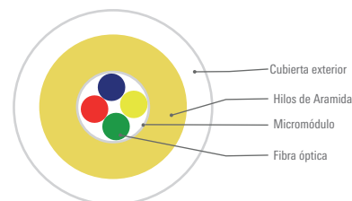
Corte de cable versión 4 fibras
